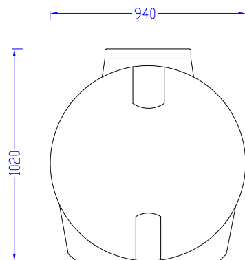
VISTA TRANSVERSAL
