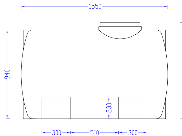
VISTA LONGITUDINAL
